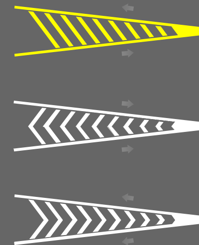
MARCAS CANALIZADORAS
